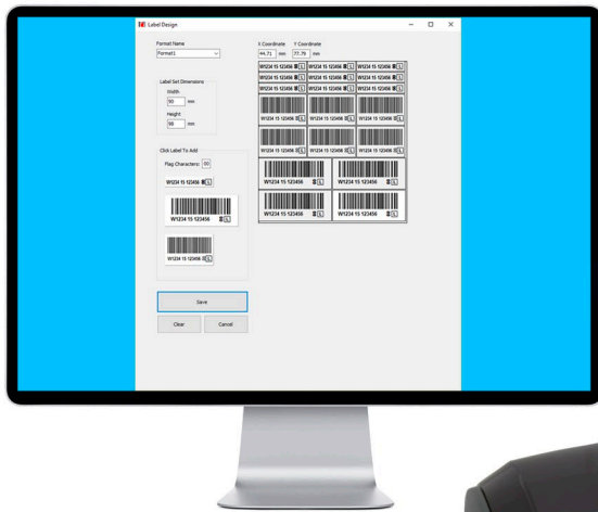
DINselect™-SA software
